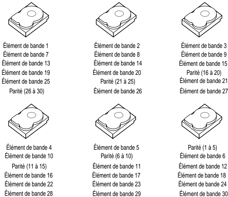
Figure 2-3. Exemple de parité distribuée (RAID 5)
